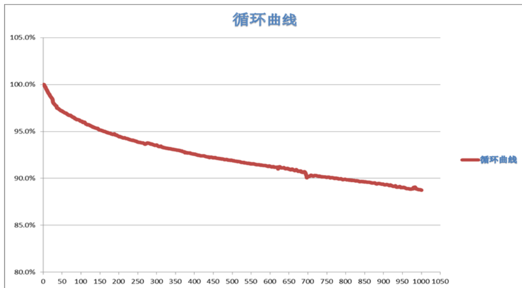
15.0Ah 磷酸铁锂电池 1C 循环曲线图 Circular curve of 15.0 Ah-LiFePO 4 cell
